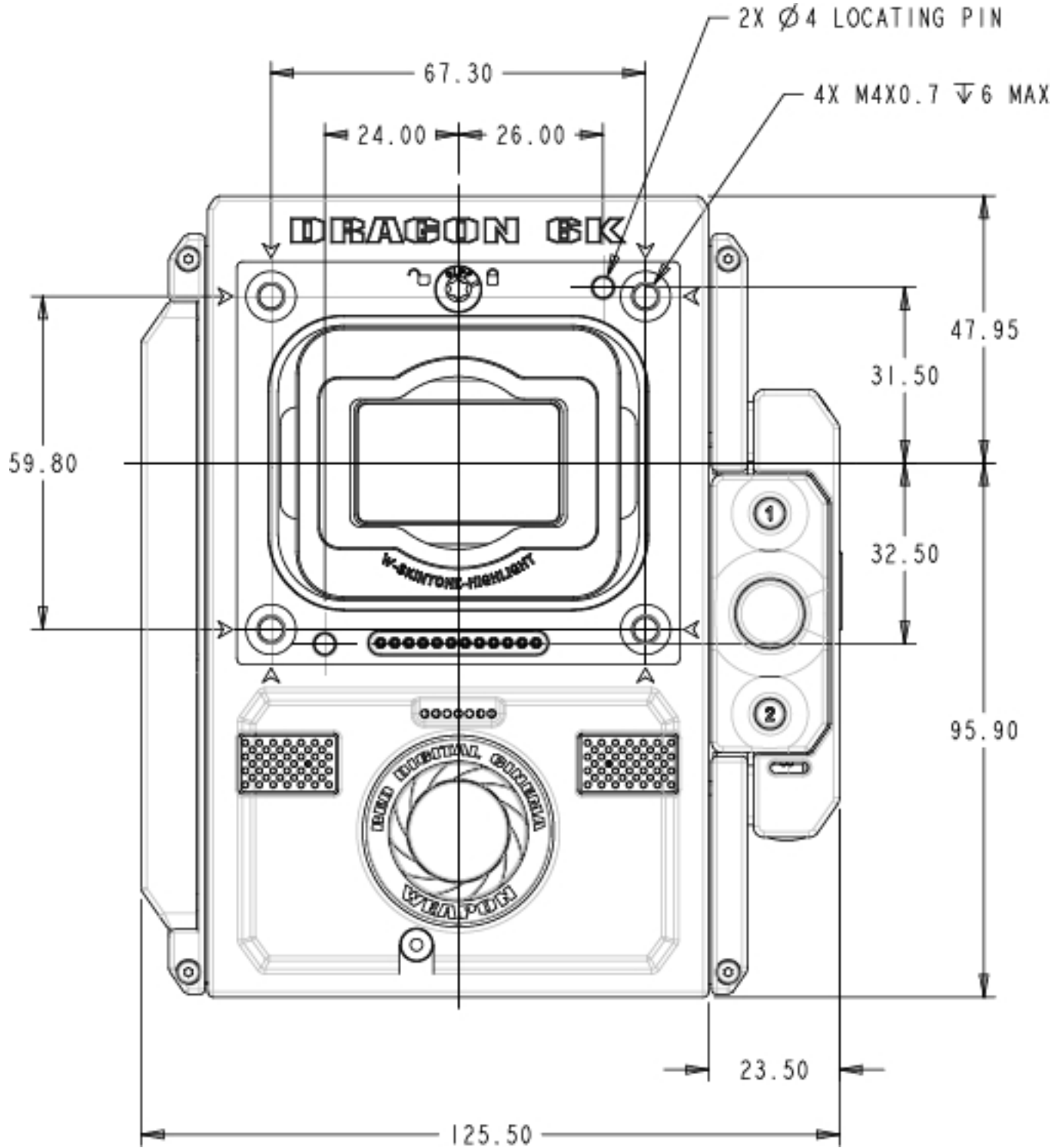
그림: WEAPON 정면도
