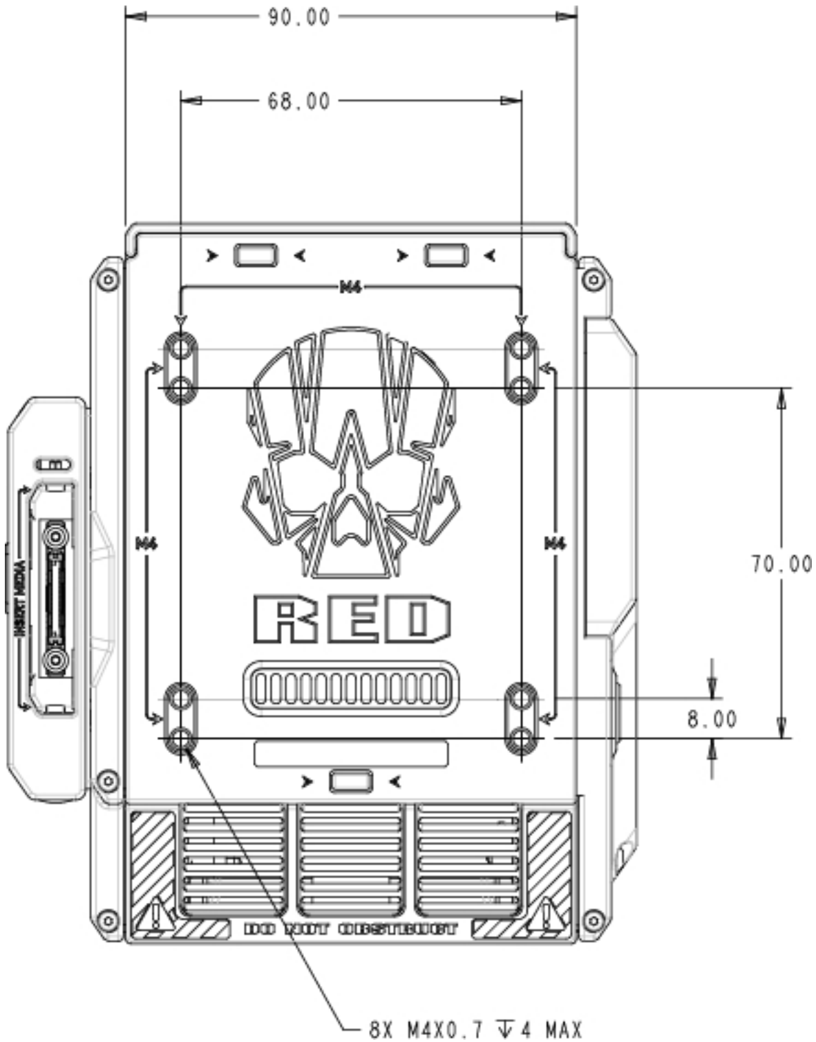
그림: WEAPON 후면도
