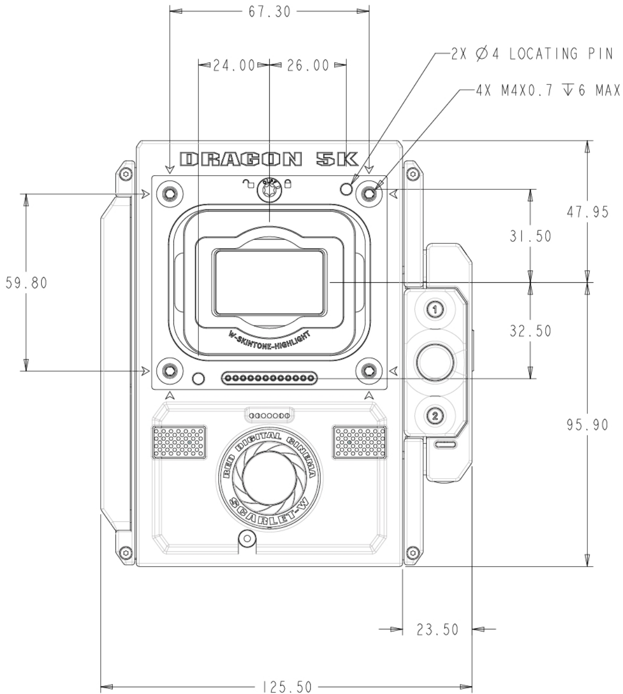
그림: SCARLET-W 정면도
