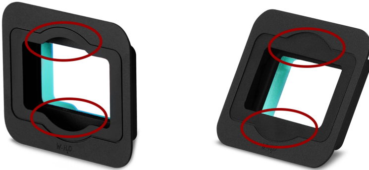
그림: 오리지널 DSMC2 OLPF, 곡선형 글래어 조리개(왼쪽); 수정 버전 DSMC2 OLPF, 직선형 글래어 조리개(오른쪽)
