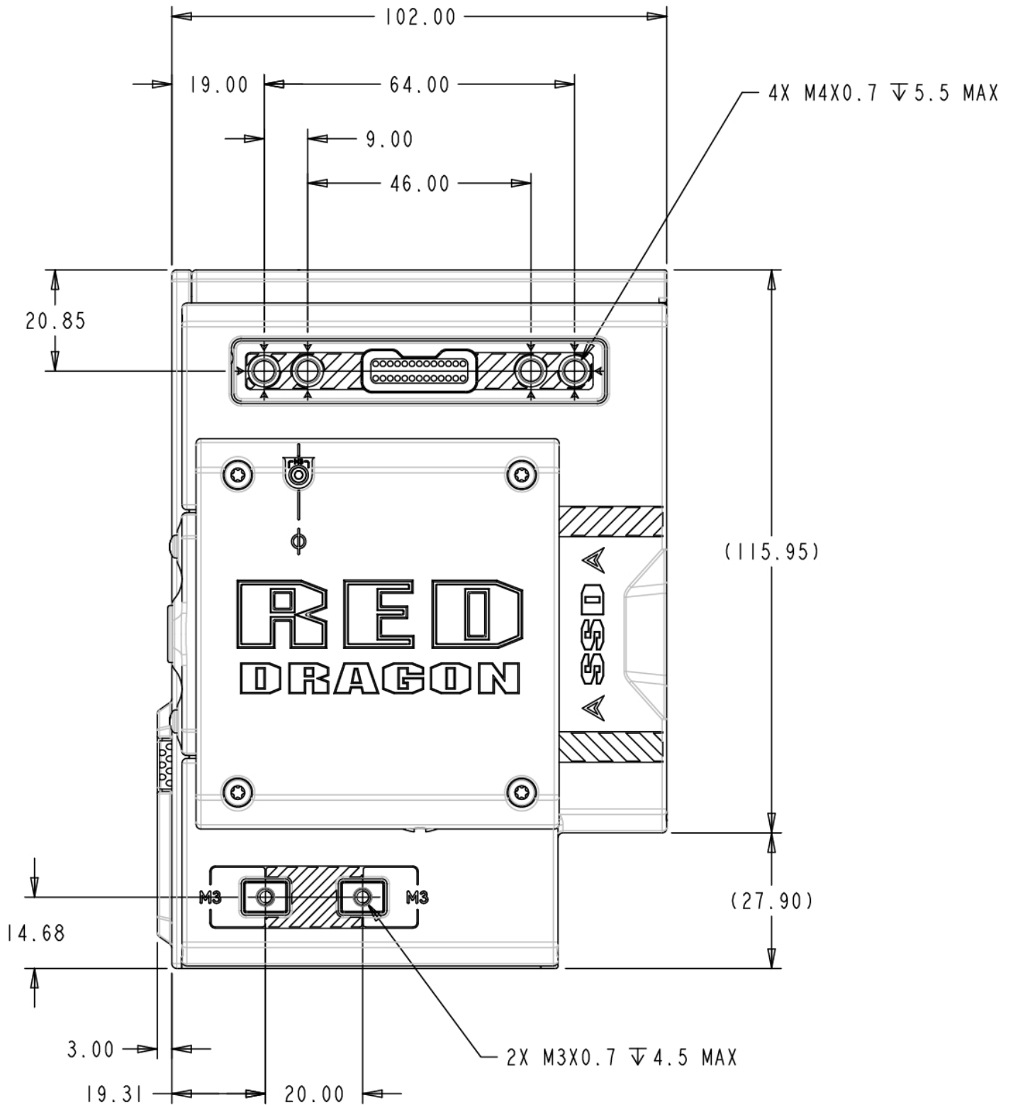
그림: WEAPON 측면도(오른쪽)
